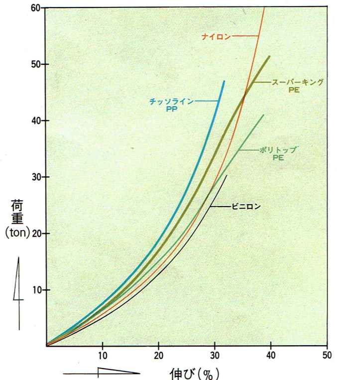
各種ロープの破断強伸度曲線 (60%ロープ)
